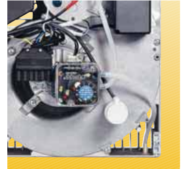
hava presostatı
